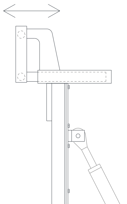
VISTA LATERALE SINISTRA
