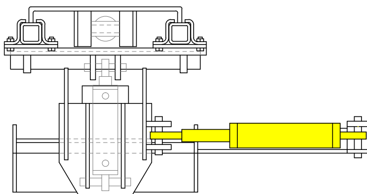
VISTA IN PIANTA
